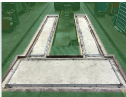
Bild: Fundamentrahmen SEP3.0+2L eingebaut
